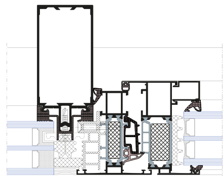
Połączenie fasady z oknem
