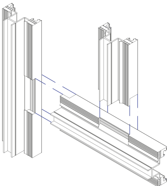
3 poziomy odwodnienia przy użyciu uszczelki płaszczowej
