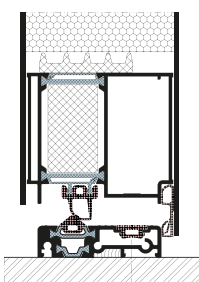
Próg aluminiowy
