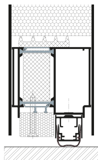
Próg opadający
