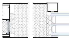
Befestigung der Verglasung
