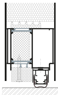
Isolierte Boden - Türdichtung
