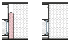
Befestigung der Füllungen
