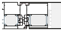
Variante mit dünnerem Paneel
